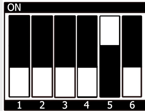
图 7: USB OTG
