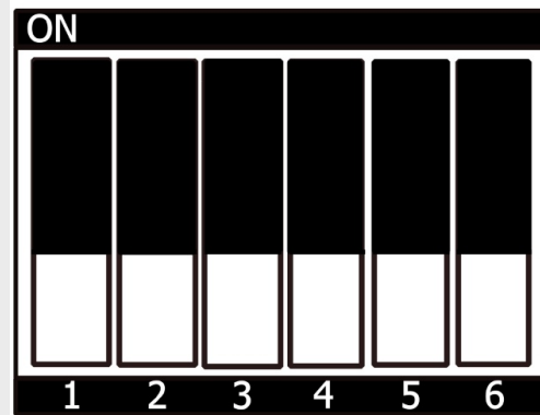
图 9: UART1 RS232
